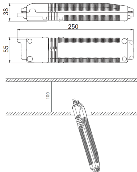
Einzelbatterie-Elektronik-Box (UH-1)
